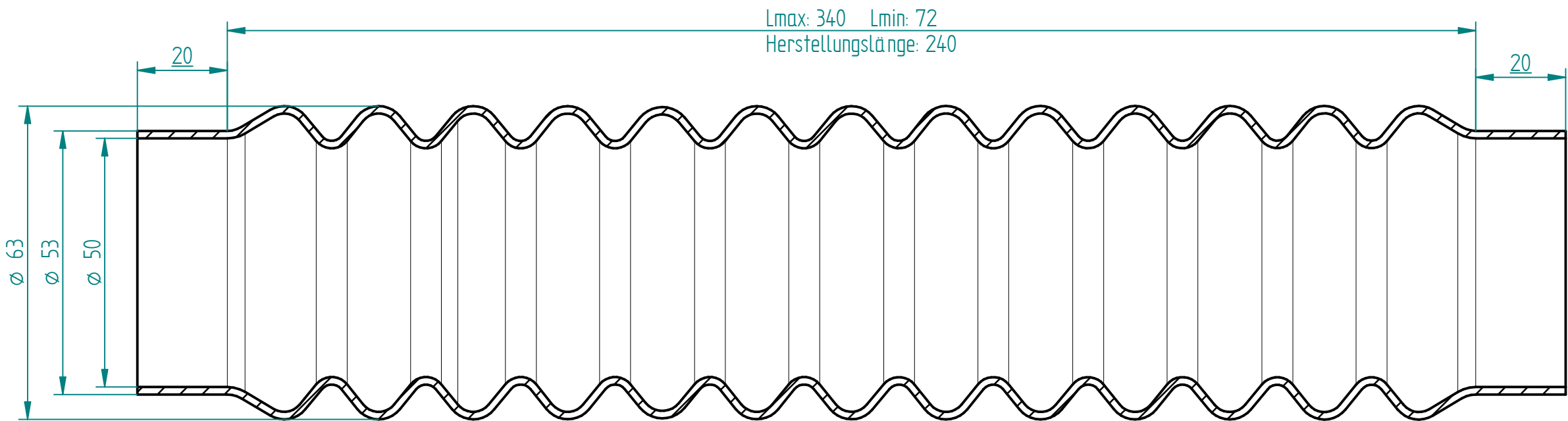
Schnitt A-A
