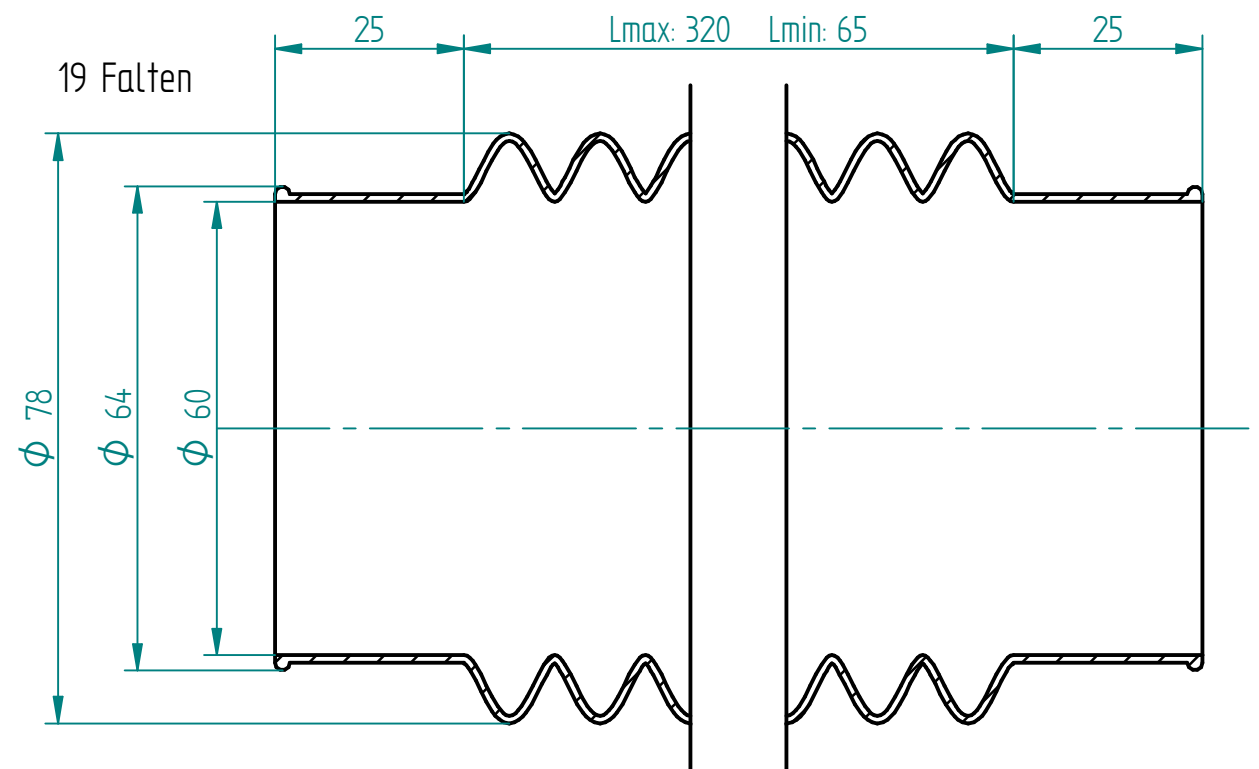
Schnitt A-A
