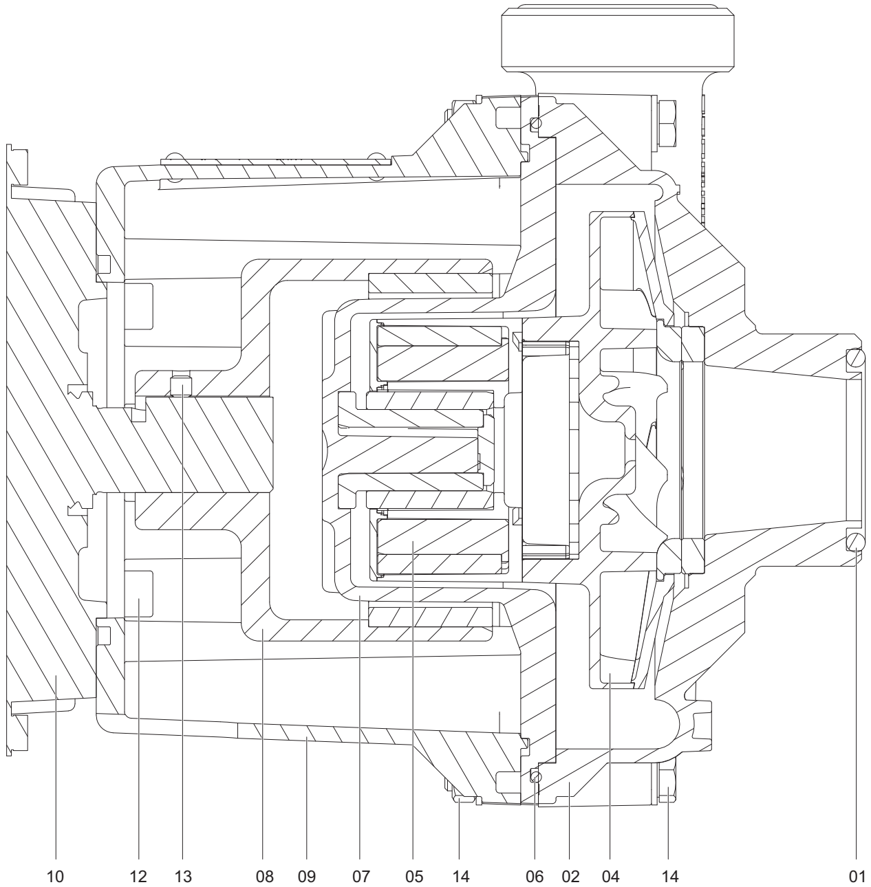
Abb. 7 Teile (Schnittzeichnung)
