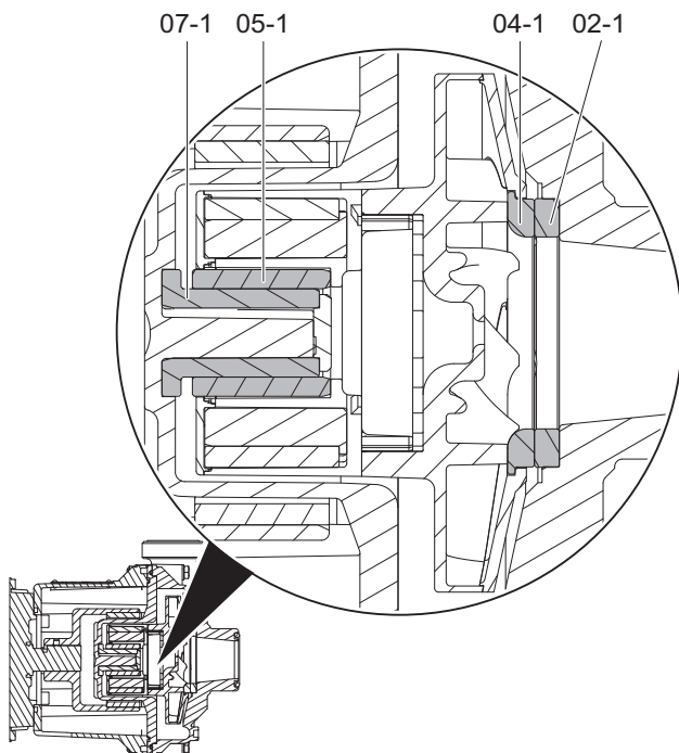
Abb. 6 Bestandteile der Gleitlager
