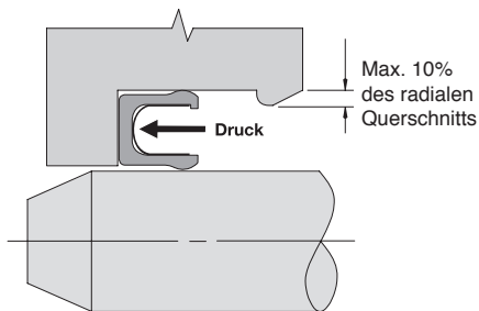
Stangendichtung Nut mit Haltenase
