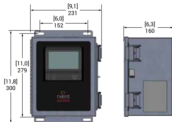
Edelstahlgehäuse mit EMR
