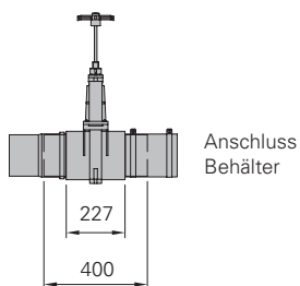
PVC-Zulaufschieber DN 150
