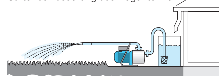
Gartenbewässerung aus Regentonnen
