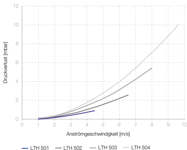
Diagramm Druckverlust LTH 500
