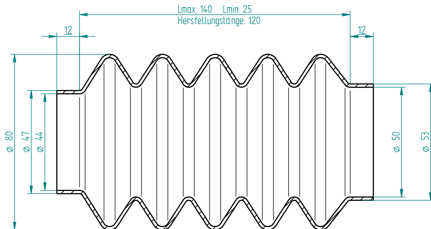
Schnitt A-A
