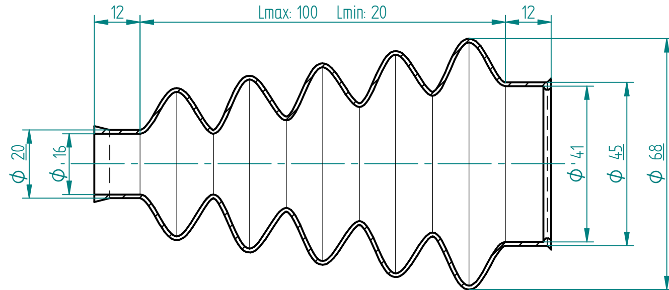
Schnitt A-A
