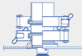
Tri-Clamp-Anschluss
