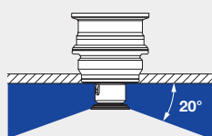
Tri-Clamp-Anschluss 1
