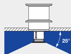
Tri-Clamp-Anschluss 2
