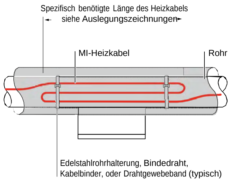
Abbildung 20: Befestigung von Schuhen und Schleifen
