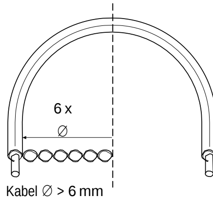
Abbildung 4: Minimaler Biegeradius von MI-Heizkabeln
