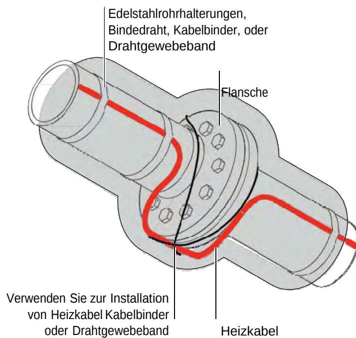
Abbildung 18: Flansche
