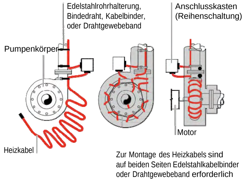
Abbildung 22: Pumpen
