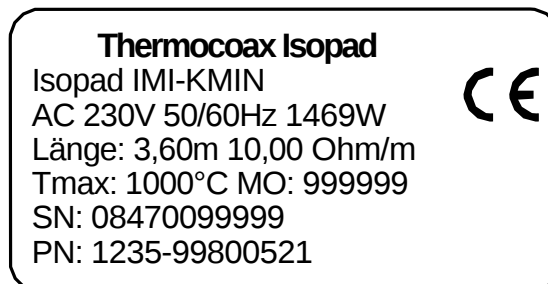
Abbildung 25: Typisches MI-Kennzeichnungsschild (Nicht-Ex-Bereiche)
