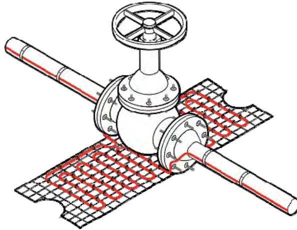
Abbildung 23: Auf Metalldrahtnetzen befestigte Kabel
