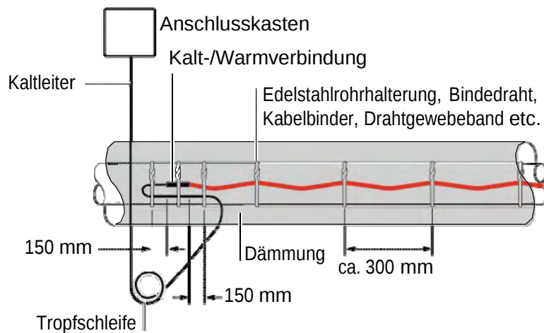
Abbildung 15: Befestigung mehrerer Heizkabel
