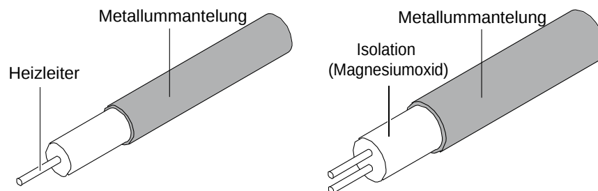
Abbildung 1: Typische Kabelbauart
