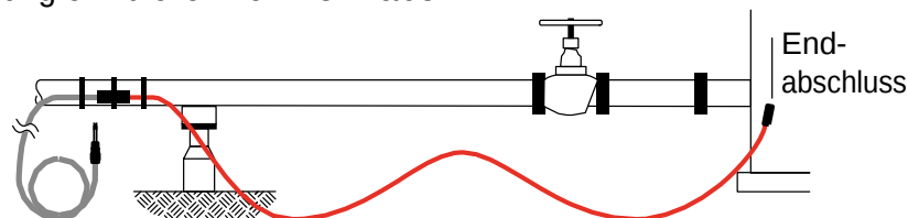
Abbildung 10: Befestigen von Kalt-/Warmverbindung und Endabschluss
