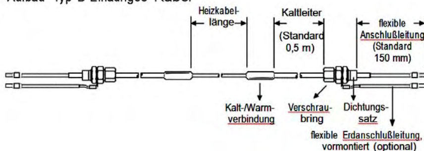
Abbildung 2: Typischer Aufbau eines Heizkabels
