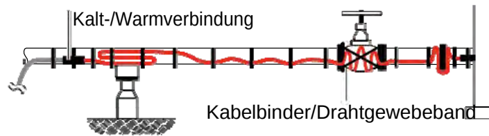
Abbildung 13: Vollständige Installation eines MI-Heizkabels
