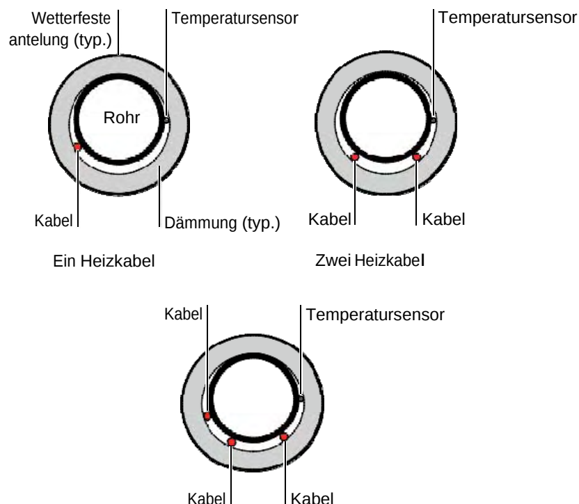
Abbildung 6: Kabelausrichtung auf Rohrleitung
