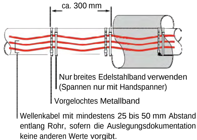
Abbildung 15: Befestigung mehrerer Heizkabel
