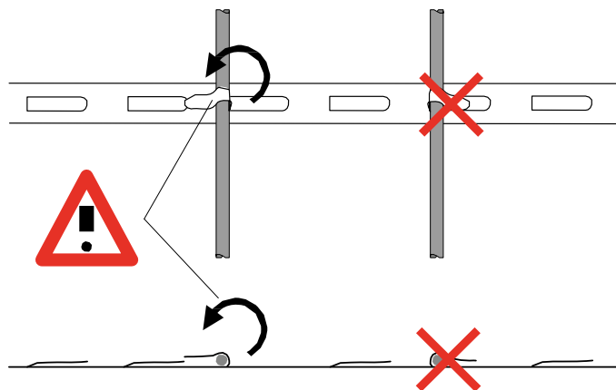
Abbildung 8: Befestigung: vorgelochtes Metallband
