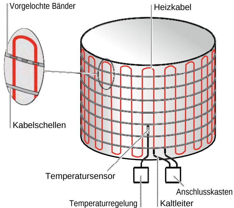
Abbildung 8: Befestigung: vorgelochtes Metallband
