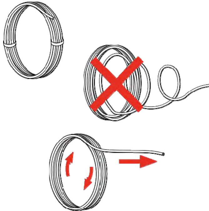
Abbildung 3: Heizkabel abrollen
