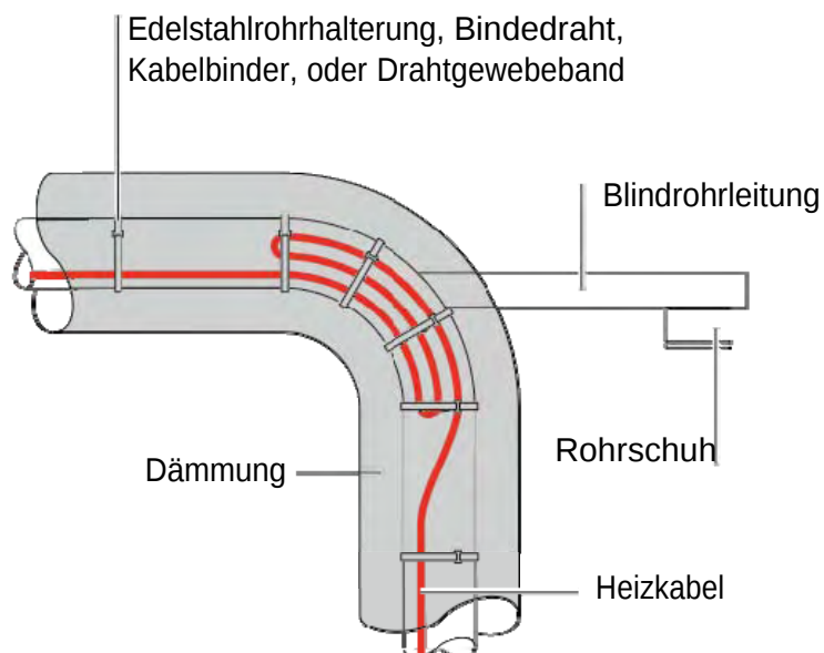
Abbildung 21: Befestigung an Blindrohren
