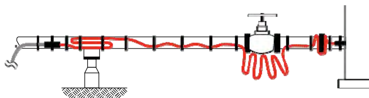
Abbildung 12: Installation von Kabeln auf Armaturen und Rohrhalterungen
