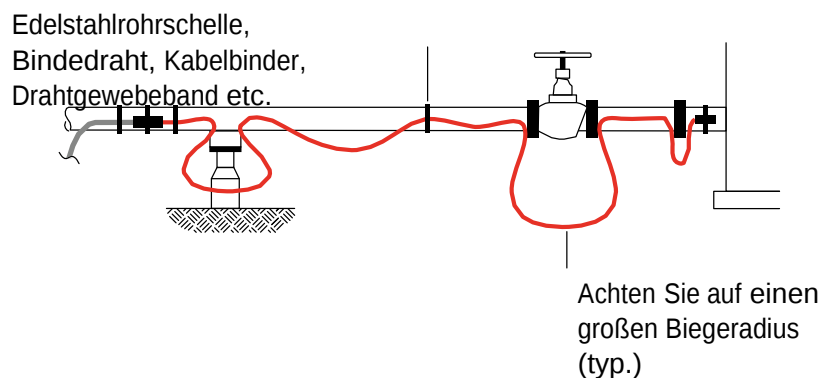
Abbildung 11: Zuschläge für Armaturen, Flansche und Rohrhalterungen
