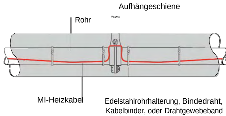
Abbildung 19: Kabelverlegung über Klemmen und Schellen
