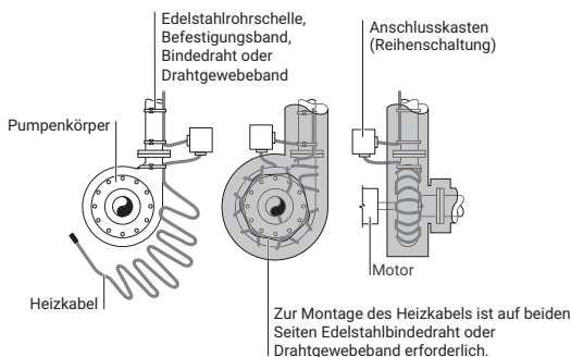
Abbildung 22: Pumpen
