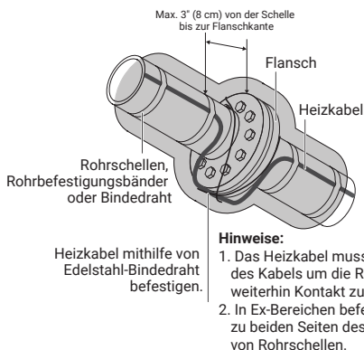
Abbildung 18: Flansche
