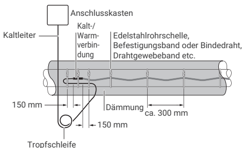
Abbildung 14: Abstand Befestigungen
