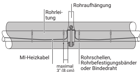
Abbildung 19: Heizkabelverlegung über Klemmen und Schellen
