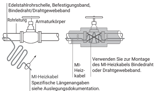
Abbildung 16b: Armaturen
